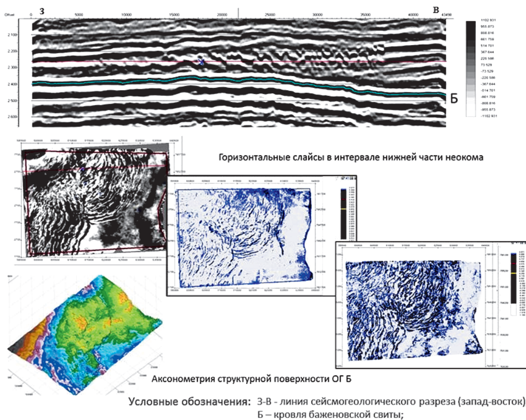
Рис. 8. Волновая картина в интервале нижней части неокома п-ова Ямал (Бородкин и др., 2018)
