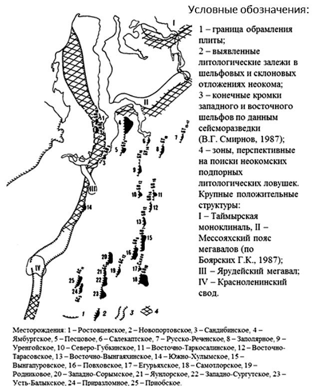
Прогнозируемые зоны распространения неокомских подпорных литологических ловушек, А.Л. Наумов, 1990 г.
