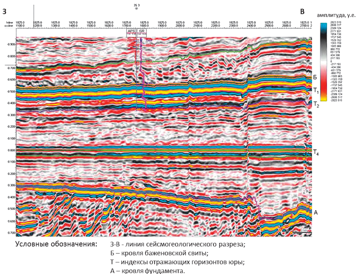
Рис. 9. Сочетание глубинного разлома с внешней границей внутриформационных деформаций (Бородкин и др., 2018)
