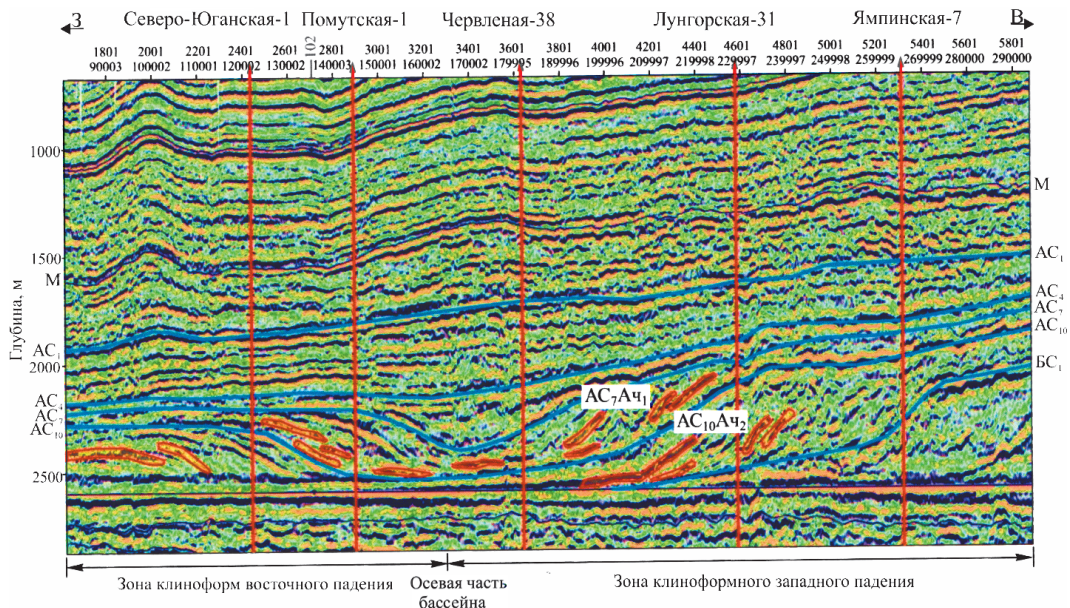
Рис. 1. Клиноформная модель неокома Западной Сибири (по данным сейсморазведки МОВ ОГТ). На сейсмическом разрезе приведены отражающие горизонты (ОГ): М – приуроченный к кровле неокомских отложений нижнего мела; AC 1 , AC 2 , AC 7 , AC 10 , BC 1 – ОГ, стратиграфически соответствующие кровле пластов
