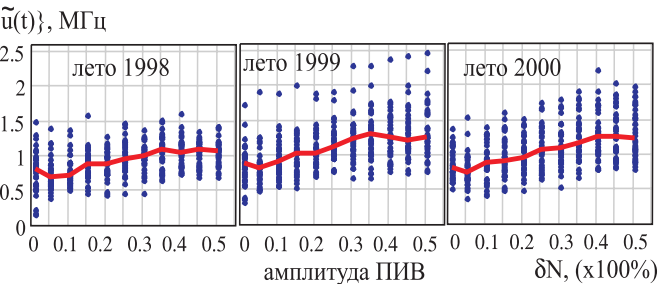
Рис. 4. Связь между амплитудой перемещающихся ионосферных возмущений и летними вариациями остаточной компоненты суточных ходов МНЧ радиолонии Кипр – Йошкар-Ола.
