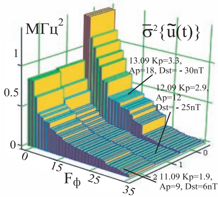
Рис. 6. Мощность остаточной компоненты суточных ходов МНЧ мода 1F трассы Инскип – Йошкар-Ола.
