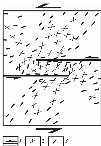
Рис. 4. Распределение вторичных сдвигов и структур растяжения во внешних зонах и внутри ступенчатого перекрытия левосторонних разломов. По данным моделирования P. Connolly, J. Cosgrove (1999). 1 – главные разломы и направление смещений по ним; 2-3 – вторичные разрывы: 2 – сдвиги; 3 – структуры растяжения.
