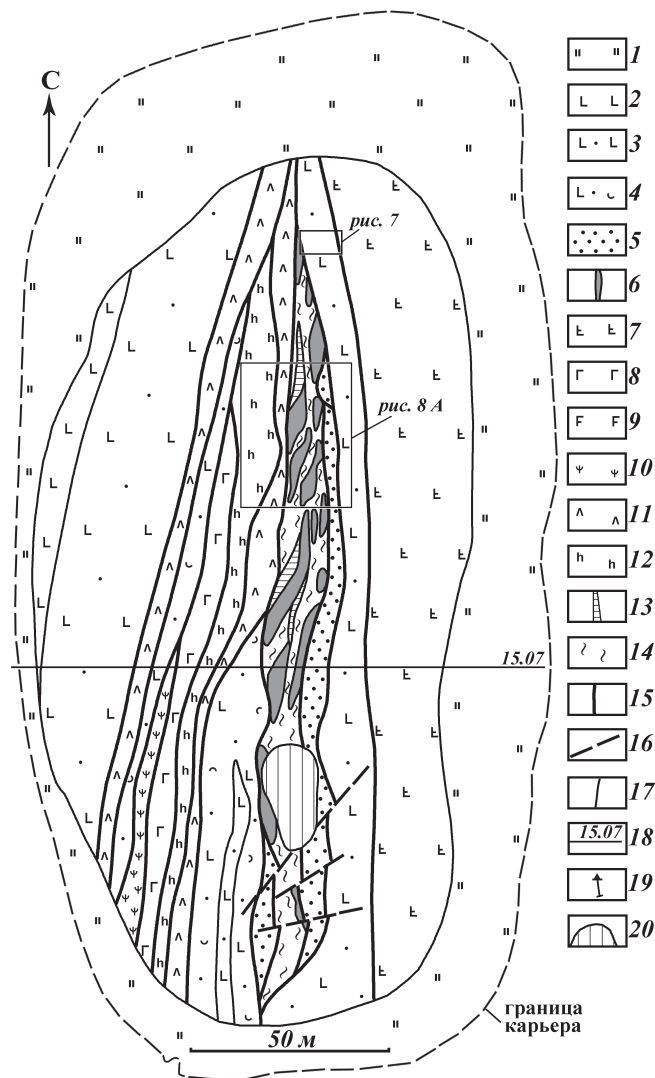
Рис. 5. Схема геологического строения карьера Ганеевского месторождения (составлена с использованием данных ЗАО НПФ «Башкирская золотодобывающая компания»). 1 – зона окисления; 2-7 – карамалыташская свита (D 2 e); 2 – базальты, 3 – туфы основного состава, 4 – туффицы основного состава, 5 – расланцованные и листовенизированные глинисто-кремнистые сланцы, туфоалевролиты, туфопесчаники и туфогравелиты, 6 – минерализованные будины кремнистых туфоалевролитов и сланцев; 7 – диабазы и их брекчии (O 2 ?); 8 – габбро и габбро-диориты; 9 – габбро-диабазы; 10 – серпентиниты; 11 – листовениты; 12 – кварц-карбонат-хлоритовые сланцы; 13 – кварцевые жилы; 14 – зоны расланцевания и смятия с глиной трения; 15 – разломы; 16 – послерудные разрывные нарушения; 17 – геологические границы; 18 – линия профиля 15.07; 19 – проекции скважин; 20 – затопленная часть карьера.
