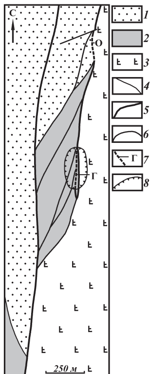
Изучением месторождения в процессе прогнозно-поисковых, поисково-разведочных и тематических работ занимались Б.Г. и С.Б. Галиуллыны, С.В. Сурин, Рис. 3. Схема геолого-структурной позиции Ганеевского месторождения (составлена с использованием данных ОАО «Башкиргеология»). 1 — вулканогенно-осадочные отложения улутауской свиты ( D_{2,3} ); 2 — вулканогенные и вулканогенно-осадочные породы карамалыташской свиты ( D_2 ); 3 — диабазы и их брекчий ( O_2? ); 4 — геологические границы; 5-6 — главные сдвиги (5) и вторичные разрывы (6), образующие дуплекс Карагайлинской разломной зоны; 7 — рудные зоны: О — Октябрьского рудопроявления, Г — Ганеевского месторождения; 8 — эксплуатационный карьер Ганеевского месторождения.
