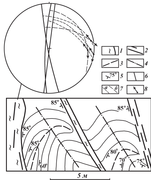
Рис. 7. Наложение поздних складок волочения F_2 на ранние складки F_1 в меридиональной разломной зоне. Диаграмма (сетка Вульфа, верхняя полусфера) векторов смещений висячих крыльев зеркал скольжения. 1 – зоны рассланцевания; 2 – зеркала скольжения; 3-4 – оси складок F_1 (3) и F_2 (4); 5 – элементы залегания; 6-8 – на диаграмме проекции на верхнюю полусферу: 6 – поверхностей зеркал скольжения, 7 – плоскостей, нормальных к поверхностям зеркал скольжения и параллельных векторам ранних (а) и поздних (б) смещений, 8 – векторов смещений висячих крыльев зеркал скольжения.
