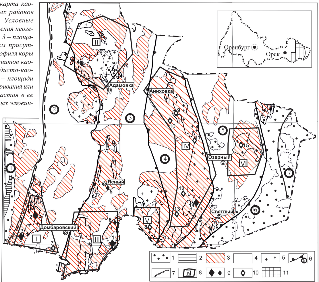
Рис. 1. Схематическая карта каолиноносности восточных районов Оренбургской области. Условные обозначения: 1 – отложения неогена; 2 – отложения юры; 3 – площади с преимущественным присутствием в верхней зоне профиля коры выветривания (Mz) элювиитов каолинового и гидрослюдисто-каолинового состава; 4 – площади отсутствия коры выветривания или же незначительного участия в ее составе выше упомянутых элювиитов; 5 – площади занятые гранитоидами и продуктами их выветривания; 6 – структурно-формационные зоны Урала: 1 – Центрально-Магнитогорская, 2 – Восточно-Магнитогорская, 3 – Кочкарско-Адамовская, 4 – Нижнесанарско-Текельдытаусская, 5 – Троицко-Буруктальская, 6 – Верхнетобольская, 7 – Айкенская; 7 – западная граница Урало-Мугоджарской каолиноносной провинции; 8 – каолиноносные районы: I – Домбаровский, II – Адамовский, III – Ушкотинский, IV – Текельдытаусский, V – Котансинский, VI – Коскольский; 9 – месторождения элювиальных каолинов: крупные и средние: 1) Южноушкотинское, 2) Домбаровское, 3) Архангельское, 14) Ковыльное; мелкие: 4) Теренсайское, 5) Киембаевское, 6) Северо-Ушкотинское; 10 – проявления элювиальных каолинов: 7) Кошенсайское, 8) Котансинское, 9) Джасайское, 10) Новое, 11) Придорожное, 12) Линейное, 13) Гостеприимное, 15) Коскольское. На врезке: 11 – Мугоджарская каолиноносная субпровинция.
