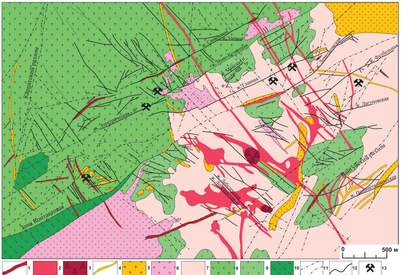
Рис. 1. Геологическая схема месторождения Дарасун (Восточное Забайкалье), построенная по материалам Дарасунской геолого-разведочной экспедиции и данным работы (Прокофьев и др., 2010), с изменениями: 1–3 амуджиканский комплекс ( J_2-K_1 ): 1 – дайки фельзитов, фельзит-порфиров, кварцевых порфиров; 2 – дарасунская каркасная интрузия (гранодиорит-порфиры, гранит-порфиры, кварцевые диоритовые порфиристы, диоритовые порфиристы); 3 – взрывные брекчи; 4 – дайки меланократовых пород ( PZ_3 ): лампрофиры, диабазы, микрогаббро, габбро-порфиристы; 5 – олекминский комплекс ( PZ_2 ): биотитовые и лейкократовые граниты, сиениты, граносиениты, кварцевые сиениты; 6, 7 – крестовский комплекс ( PZ_1 ): 6 – диориты, кварцевые диориты; 7 – биотит-роговообманковые гранодиориты; 8–10 – кручининский комплекс ( PZ_1 ): 8 – гранитизированное и амфиболитованное габбро, 9 – габбро, габбро-диориты, 10 – оливковое габбро, пироксениты, троктолиты; 11 – тектонические нарушения; 12 – рудные жилы; 13 – шахты. Подписаны крупные жилы.
