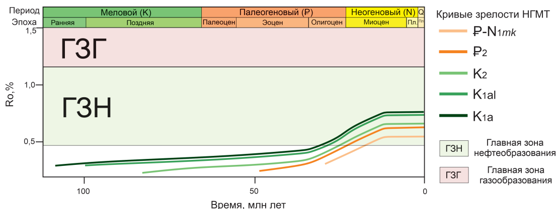
Рис. 10. Катагенетическая преобразованность нефтематеринских пород от времени ( R_o , %) в пределах Азово-Майкопской системы поднятий
