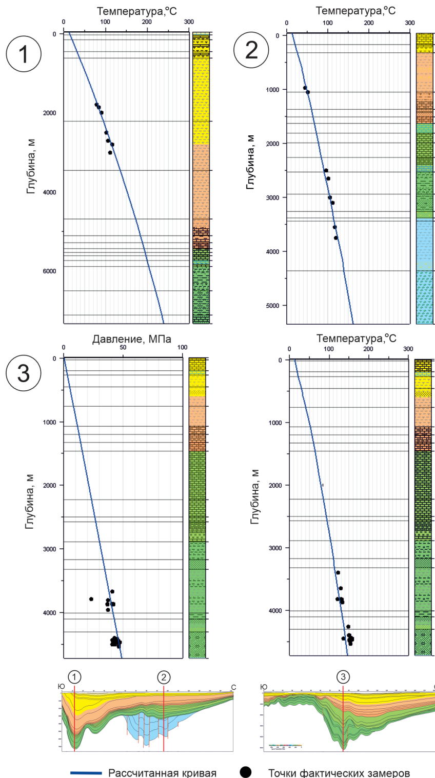
Рис. 6. Калибровочные графики соответствия замеренных температур и давлений, снятых со скважин Индоло-Кубанского (1) и Сивашского прогибов (2, 3), расчетным показателям модели (по (Богаец и др., 1973))
