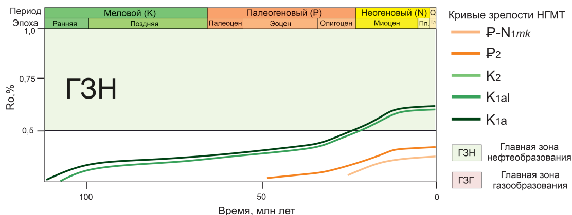
Рис. 11. Катагенетическая преобразованность нефтематеринских пород от времени ( R_o , %) в пределах западной Молдавско-Северо-Черноморской системы прогибов (в районе профиля I-I')
