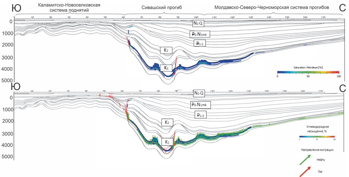
Рис. 13. Результаты моделирования профиля I-I': на верхнем профиле показано углеводородное насыщение (%); на нижнем – направление миграции углеводородов (положение профиля показано на рис. 3)
