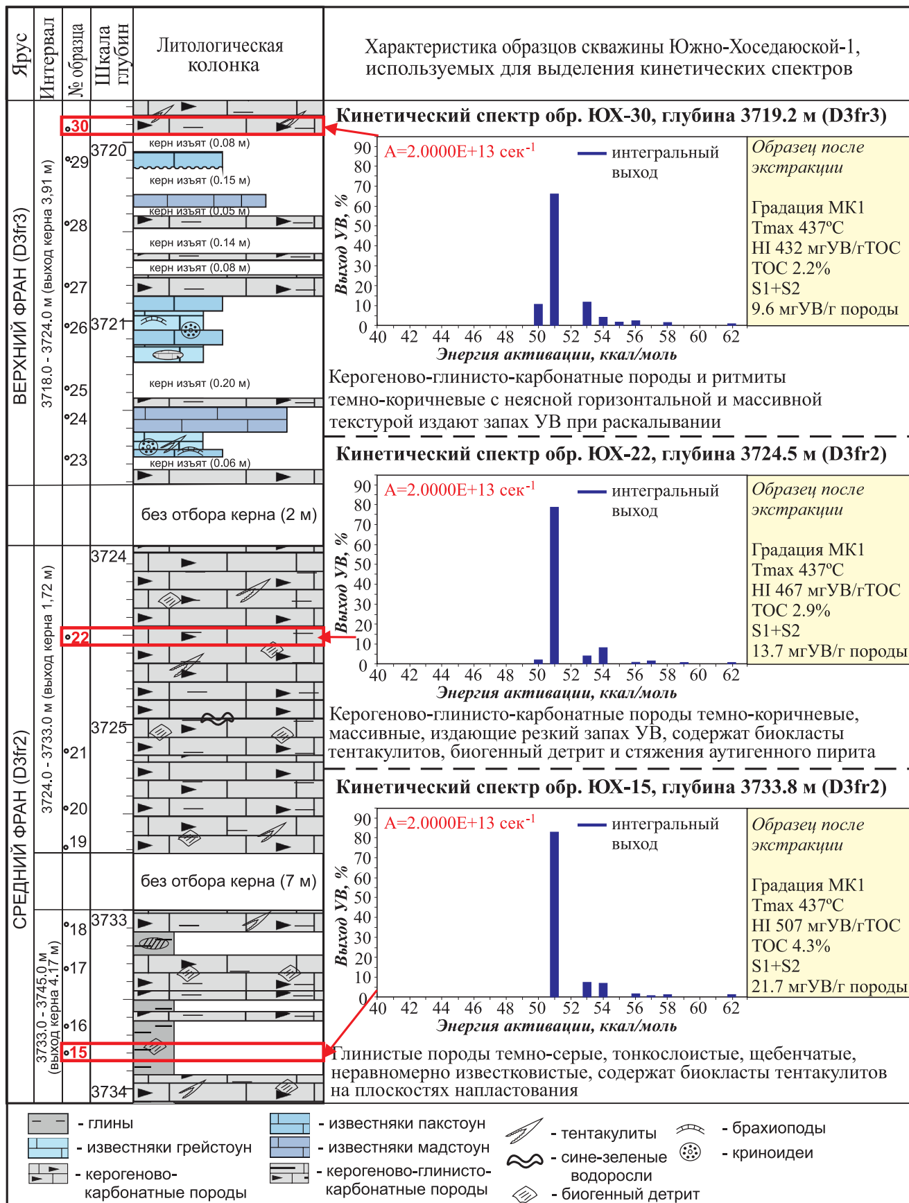
Рис. 5. Кинетические спектры деструкции керогена доминирующих отложений в разрезе скважины Южно-Хоседаюская-1
