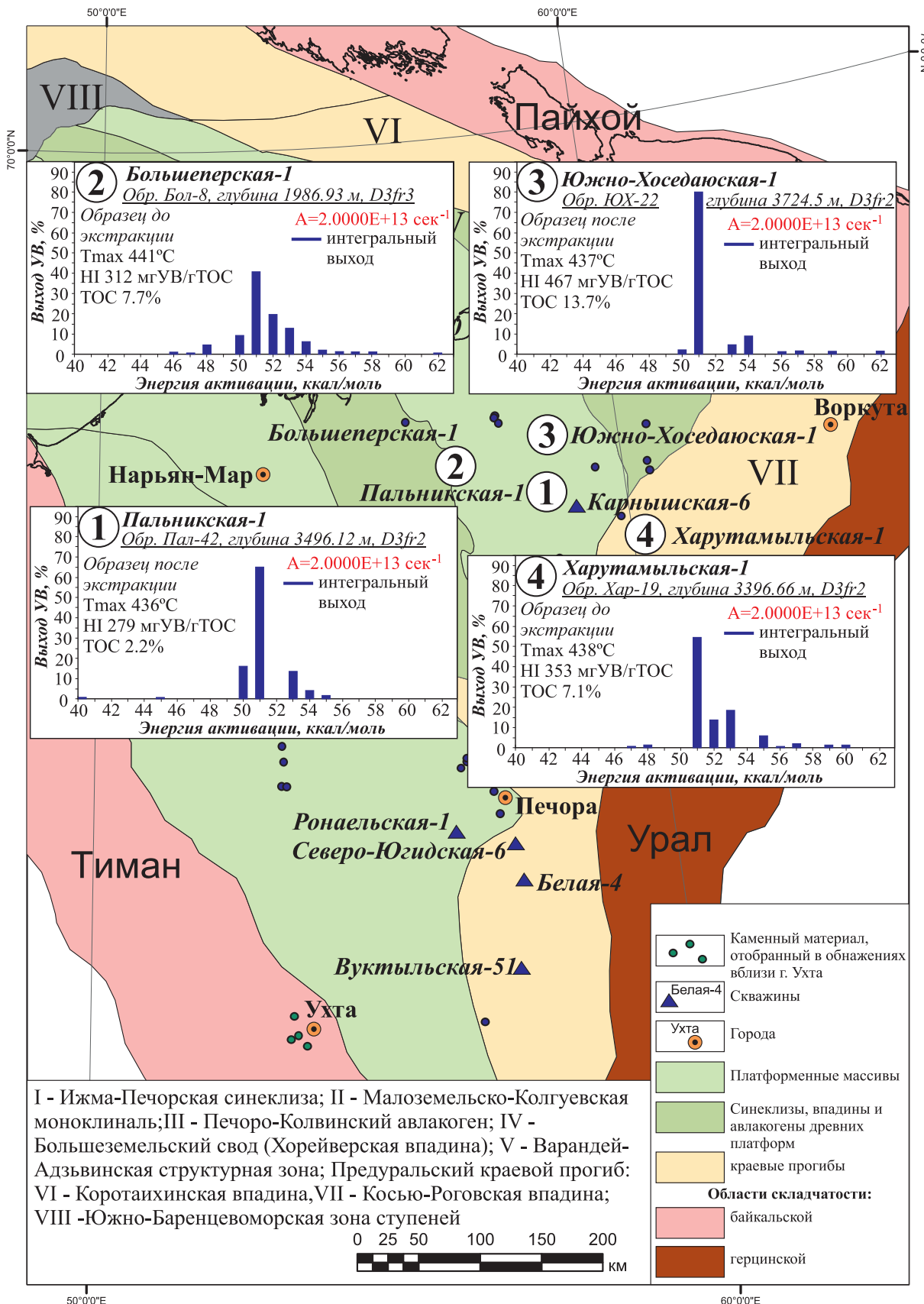
Рис. 7. Вариации кинетических спектров разрушения керогена доманиковых отложений ТПНГБ (в Хорейверской впадине и Предуральском краевом прогибе)
