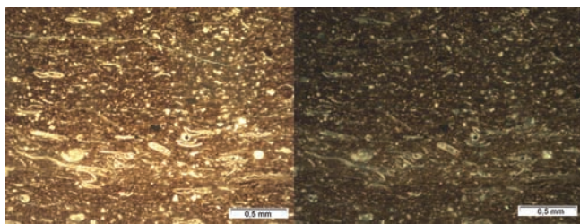
Рис. 12. Глинисто-карбонатная порода с биокластами тентакулитов. Сквжина Пальникская, образец 49. Фото шлифа: николи параллельные, скрещенные.
