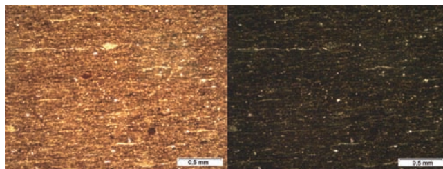
Рис. 14. Аргиллит. Сквжина Пальникская, образец 53. Фото шлифа: николи параллельные, скрещенные.
