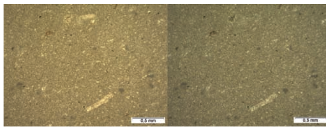
Рис. 13. Известняк (мадстоун). Сквжина Пальникская, образец 52. Фото шлифа: николи параллельные, скрещенные.
