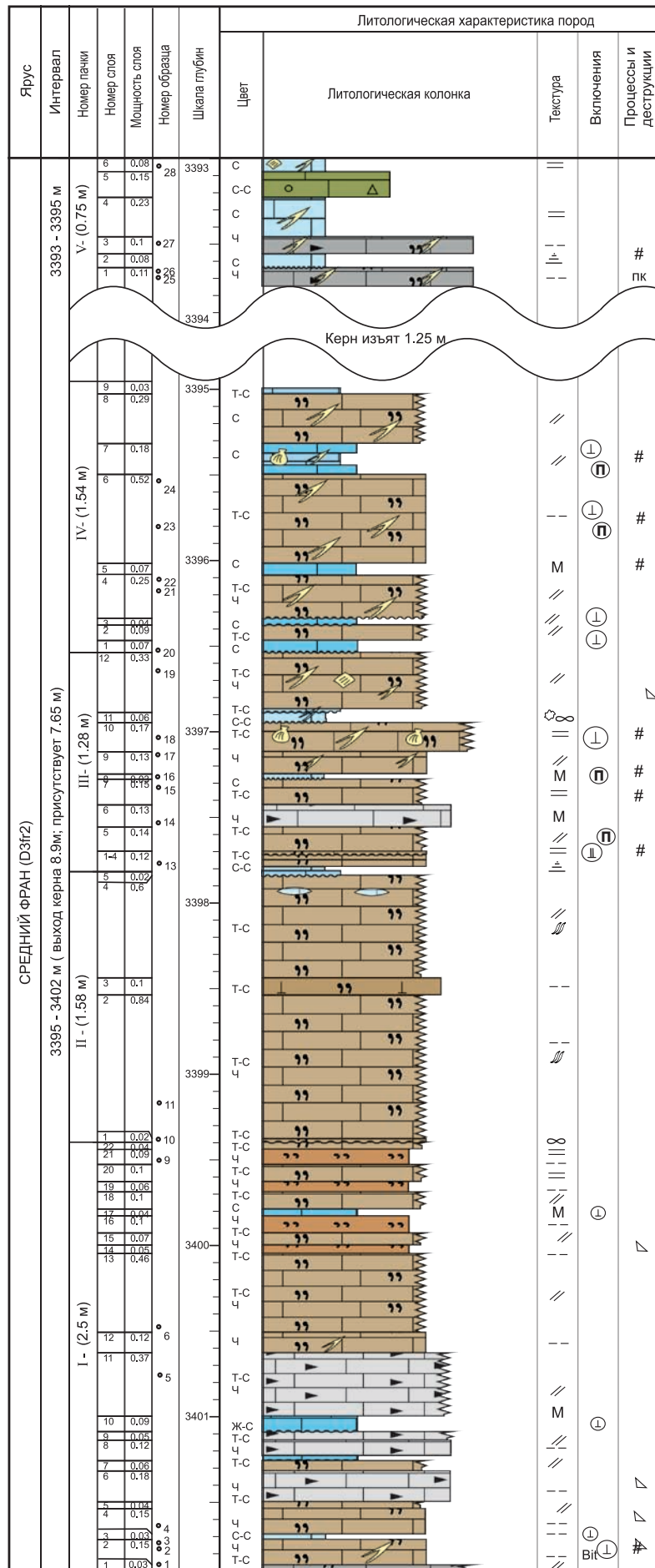
Рис. 5. Литологический разрез скв. Харутамылькская. Средний фран. Условные обозначения на рис. 6.
