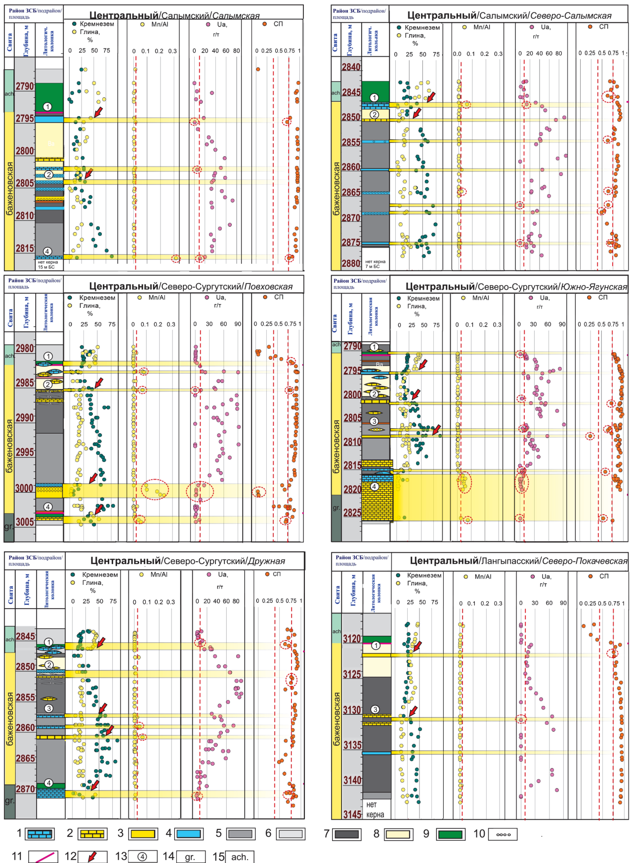
Рис. 2. Литологические колонки и диаграммы распределений по разрезу кремнезема и глинистого материала, значений редокс показателей (СП, U_a , Mn/Al) в породах баженовской свиты и зон ее перехода во вмещающие отложения Центрального района ЗСБ. 1 – доломиты породы и доломитовые микститы, 2 – известняки и известковые породы, 3 – известковистые микститы, 4 – доломитистые микститы, 5 – силициты, 6 – микститы глинистые и аргиллиты, 7 – микститы кероген-глинисто-кремнистые, 8 – микститы кероген-кремнисто-карбонатные с реликтами кокколита, 9 – пиритовые низкоуглеродистые породы, 10 – апорадиолариты, 11 – границы баженовской свиты; 12 – стрелки указывают на границы изменения вещественного состава пород, 13 – геохимический барьер, 14 – георгиевская свита, 15 – ачимовская толща.
