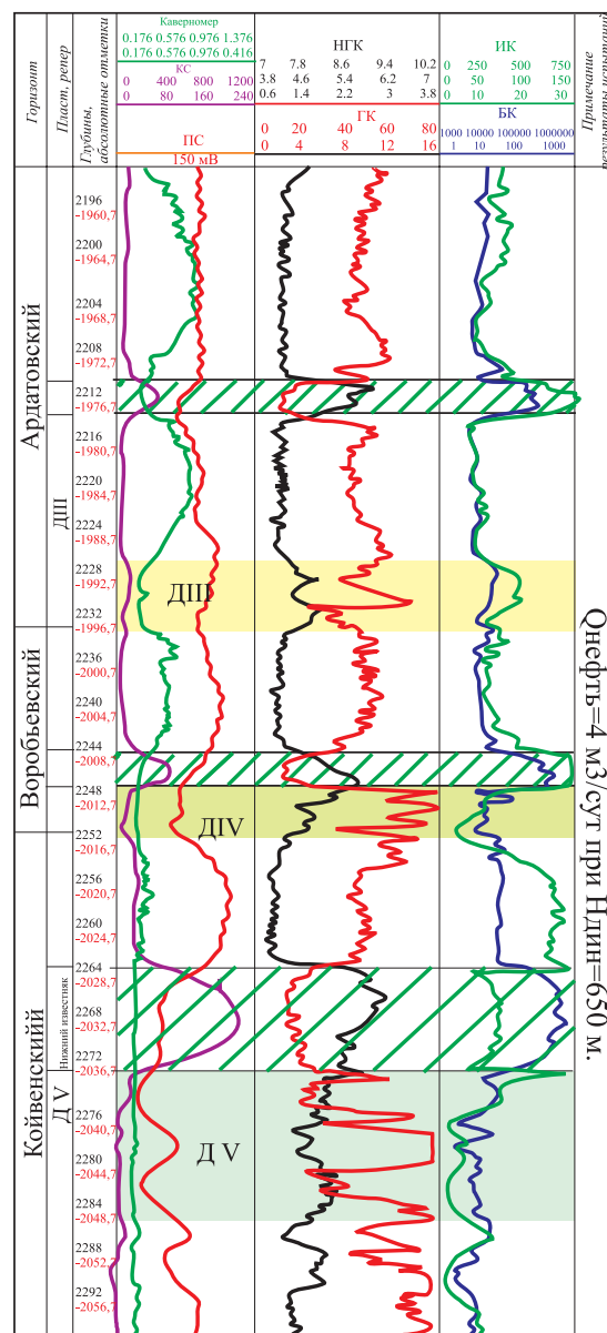
Рис. 2. Фрагмент короткодиаграммы терригенной девонской толщи на Исайкинской площади.
