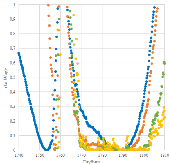
Рис. 6. Отклонение от среднего значения для вронскиана по глубине, где шифр кривых – это степень сглаживания термограммы
