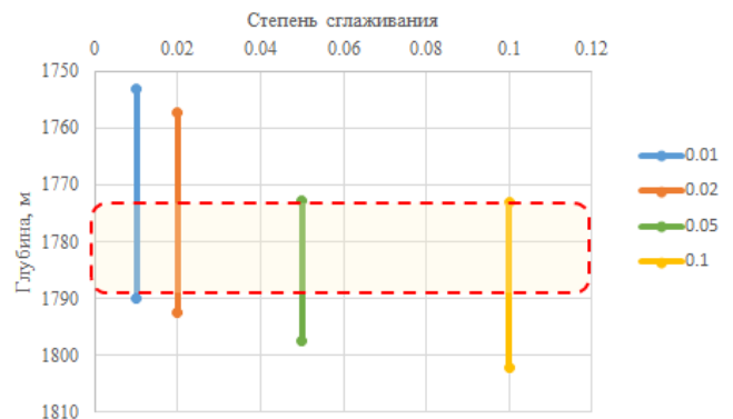
Рис. 7. Интервалы по глубине прогнозного линейного тренда, где шифр кривых – это степень сглаживания термограмм
