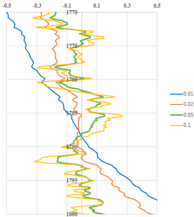
Рис. 5. Вид вронскиана по глубине, шифр кривых – это степень сглаживания
