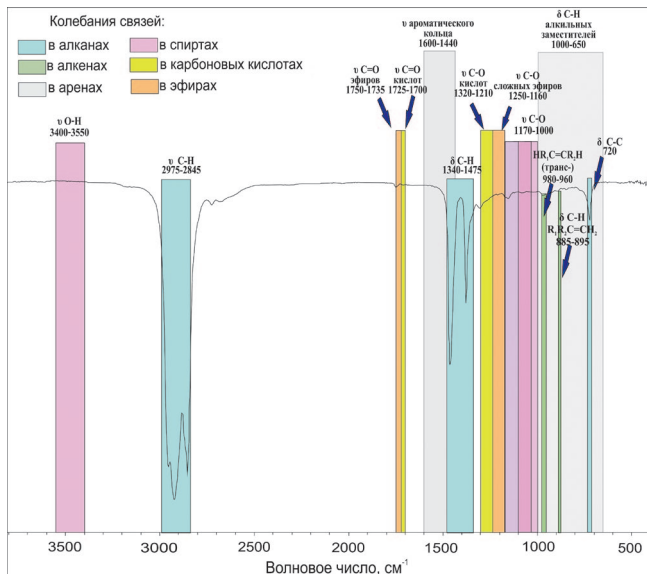
Рис. 6. Валентные ( \nu ) и деформационные ( \delta ) колебания различных связей, нанесённые на ИК-спектр вазелинового масла
