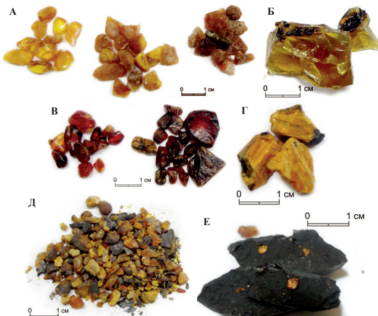
Рис. 4. Макрофотографии образцов янтарей и ископаемых смол, исследованных в работе: А – Балтийский янтарь (Калининградская обл.) (Pg 2 ), Б – Малайзия (N 1 ), В – о.Сахалин, месторождение Стародубское (Pg 2 ), Г – Центральная Европа (валховит) (K 2 ), Д – образцы янтаря (север Якутии) (Pg 2 ), Е – бурый уголь с зернами янтаря, север Якутии (Pg 2 )
