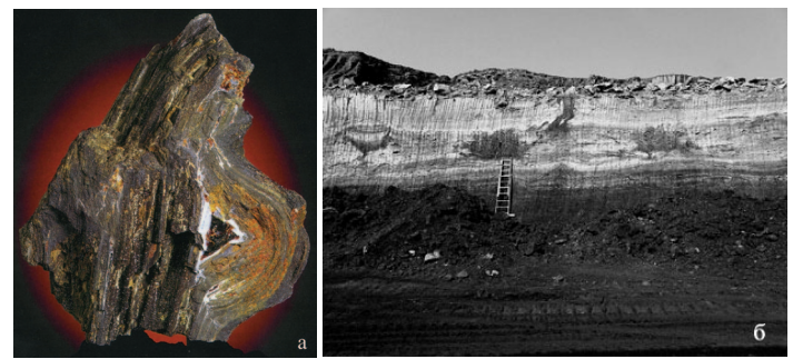
Рис. 2. Мостецкий буроугольный бассейн (Чешская Республика). а – «Капля» дуксита, размером до 25 см, в минерализованной части древесины ископаемых пней; б – «Пеньковый горизонт» в разрезе угольного карьера Билина
