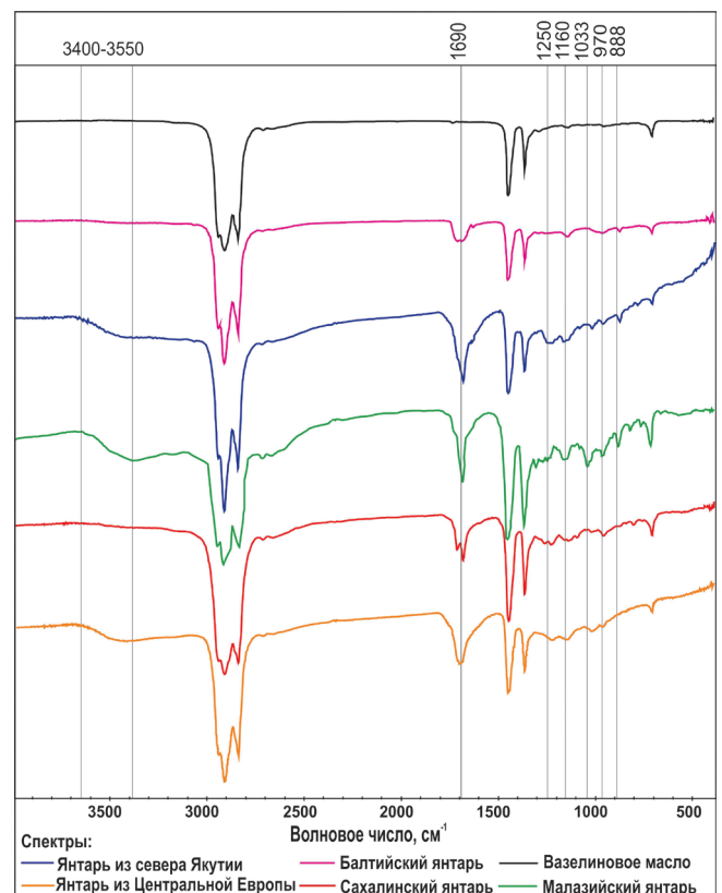
Рис. 8. Изображение ИК-спектров исследованных образцов янтарей
