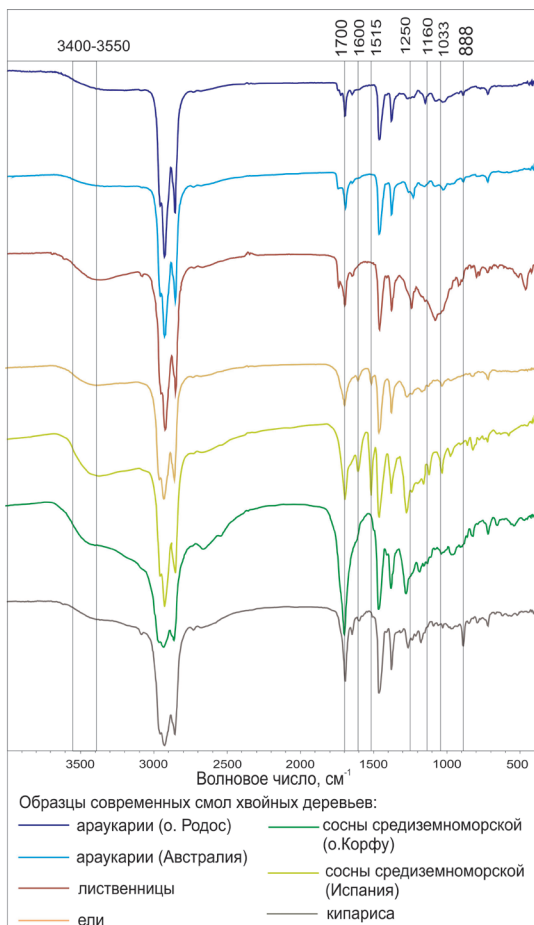
Рис. 9. Изображение ИК-спектров исследованных образцов смол современных хвойных растений
