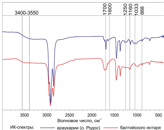
Рис. 10. Сравнение ИК-спектров Балтийского янтара и смолы араукарии
