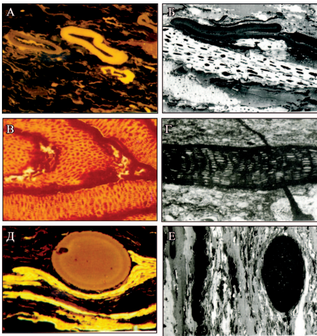
Рис. 1. Фототаблица (левая колонка – проходящий свет, правая колонка – отраженный свет): А, Б – споринит, Б – споринит – темный, фузениит – светлый; В, Г – суберинит; Д, Е – резинит (округлый), кутинит (удлиненный) (Atlas..., 1996)
