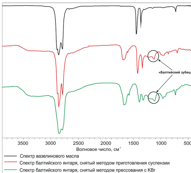
Рис. 7. Сравнение ИК-спектра вазелинового масла, ИК-спектра, полученного методом прессования с KBr и ИК-спектра, полученного методом суспензии
