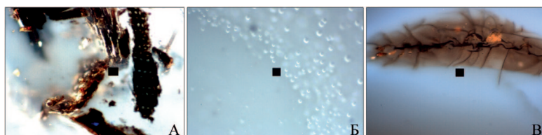
Рис. 5. Фотографии анилифов (фото Н.В.Прониной) янтарей Балтийского региона (А, Б) и о.Сахалин (В): А – янтарь коричневый. В основной массе включения растительных тканей с клеточной текстурой; Б – янтарь светло-желтый. Пузырьки предположительно воздуха и воды; В – янтарь Стародубского месторождения. Трещины заполнены, возможно, битумом
