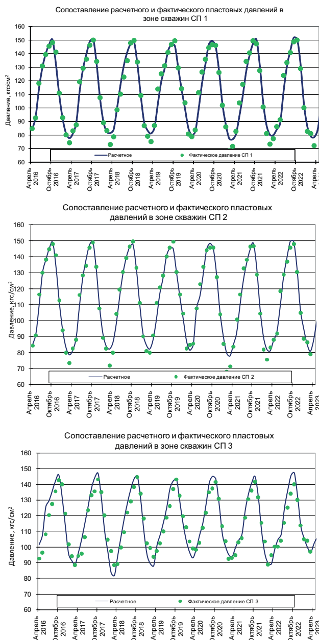
Рис. 2. Сопоставление средних расчетных и контролируемых пластовых давлений по зонам СП 1, СП 2, СП 3, Н 37 и во 2-м объекте
