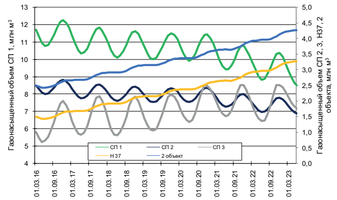
Рис. 3. Динамика расчетных газонасыщенных поровых объемов по зонам СП 1-го объекта и во 2-м объекте
