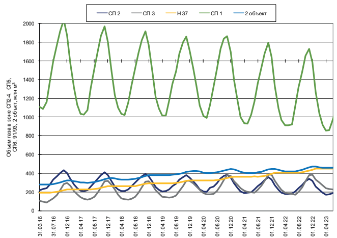
Рис. 4. Динамика расчетных объемов газа по зонам 1-го объекта и во 2-м объекте
