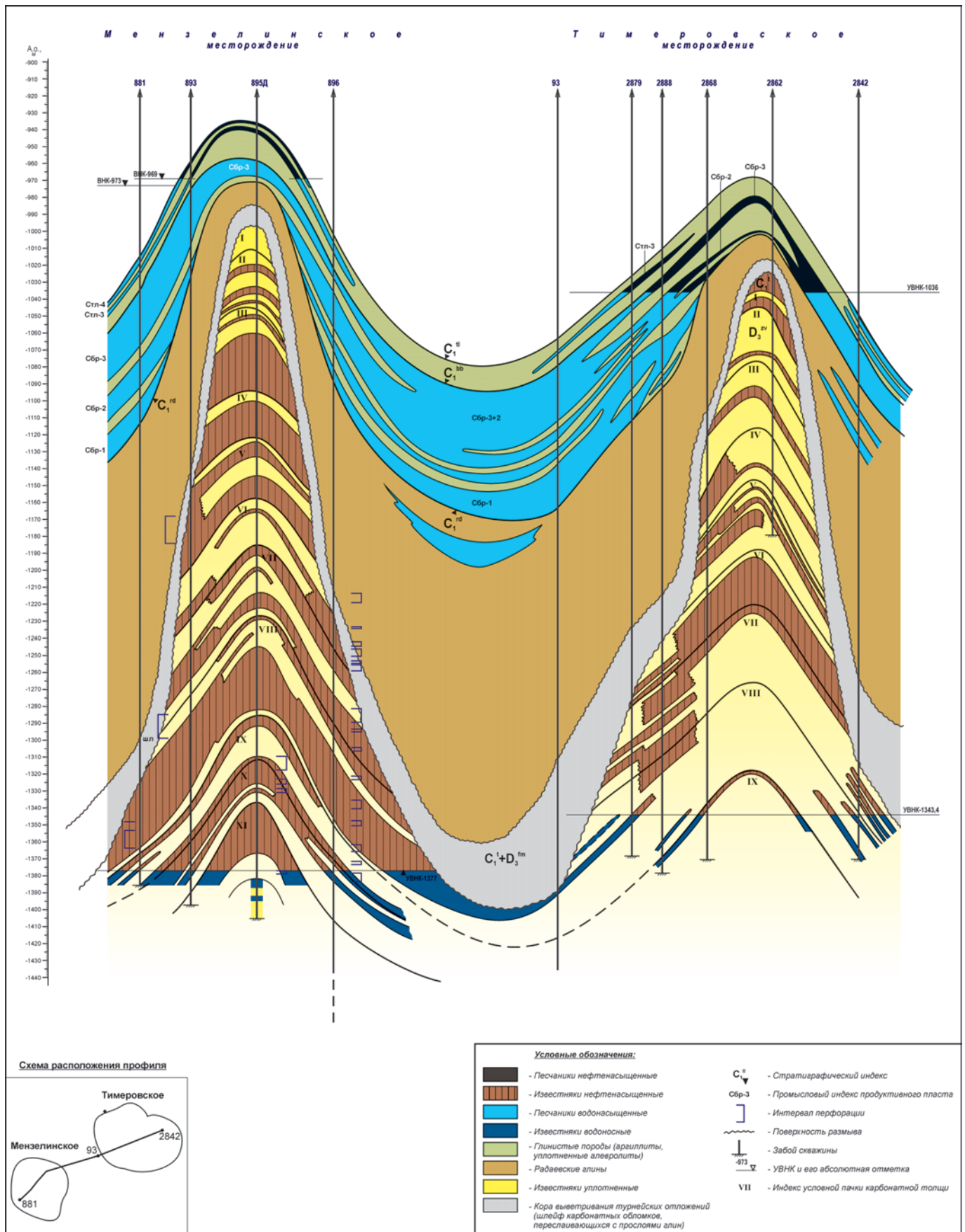
Рис. 4. Схематический геологический профиль нижнекаменноугольно-верхнедевонской толщи по скважинам Мензелинского и Тимеровского месторождений
